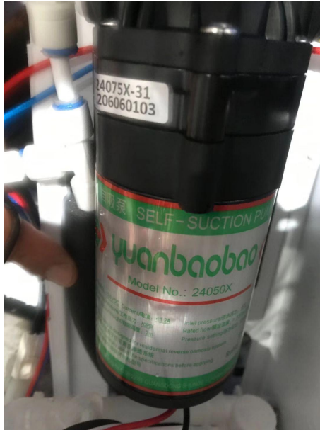
增压泵
